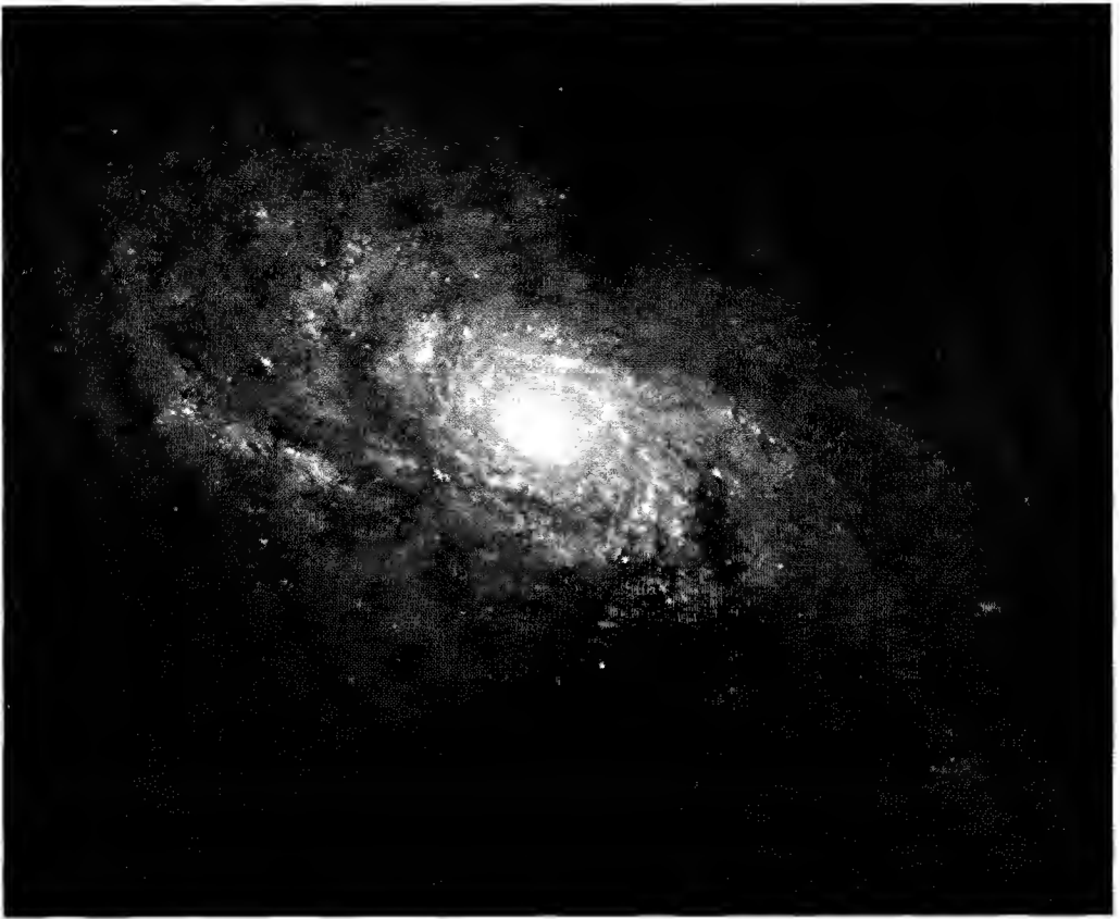
صورة لإحدى المجرات وهي تشبه مجرتنا درب اللبانة
